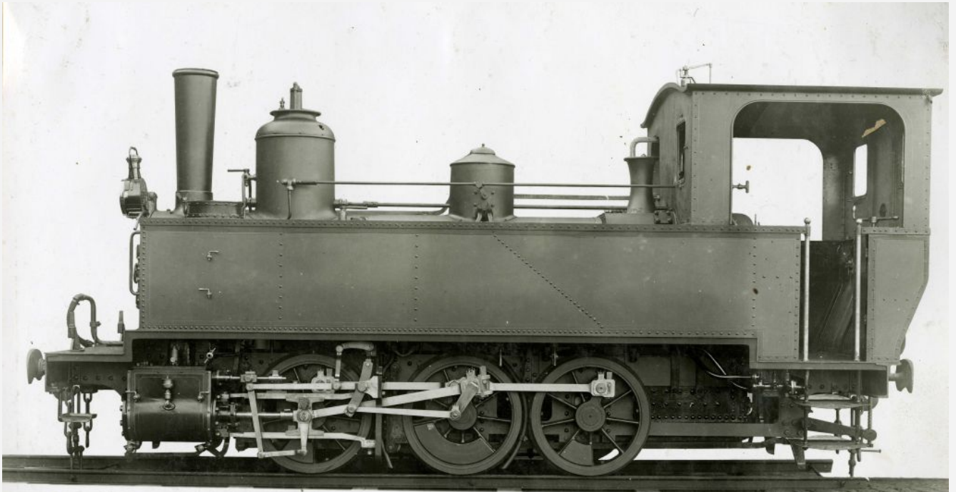
Tubize 955-974 de 1895 (BM114-133) pour le CF d'intérêt local de l'Anjou (n° 51-70). Photographie d'usine, coll. Musée 'de la Porte' à Tubize.
